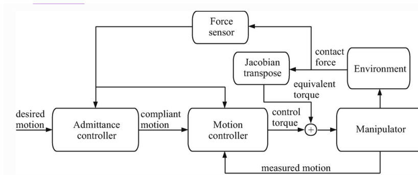
FIGURE II.1.24 – Schema qui illustre le fonctionnement de l'admittance. Source : le livre[0]
