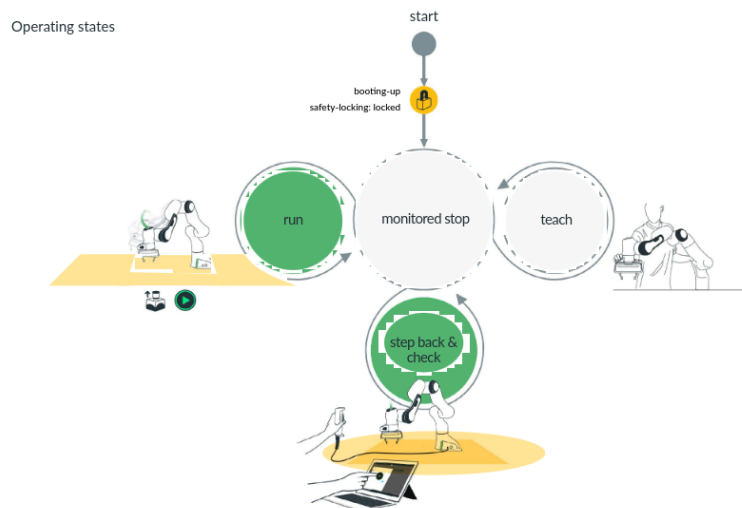
FIGURE III.1.21 – Fonctionnement du mode apprentissage pour le bras robotique Panda. Source : FRANKA EMIKA ROBOT'S INSTRUCTION HANDBOOK
