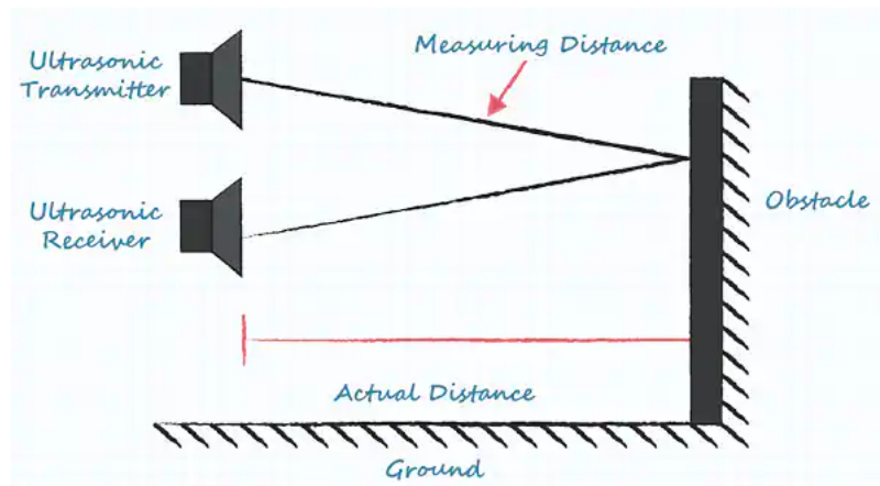
FIGURE III.1.12 – Exemple de calcul de la distance entre un émetteur et un récepteur à ultrasons. Source de l'image : CUI Devices
