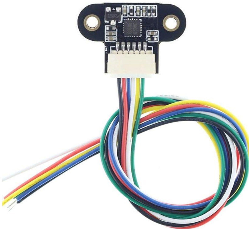
FIGURE III.1.13 – Capteur TOF10120, dont la distance couverte est entre 5cm et 180cm.
