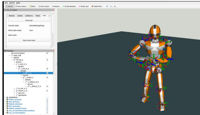
FIGURE III.1.33 – Still de la simulation avec le costume XSens dans Rviz.
