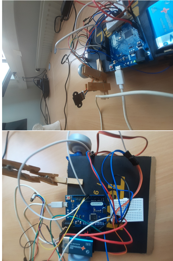
FIGURE III.1.14 – La dernière phase du prototype, avant la résidence pratique
