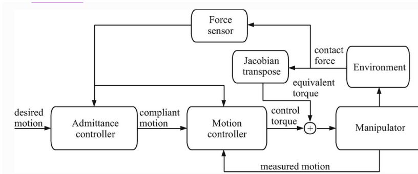
FIGURE III.1.22 – Schema qui illustre le fonctionnement de l'admittance. Source : le livre[0]
