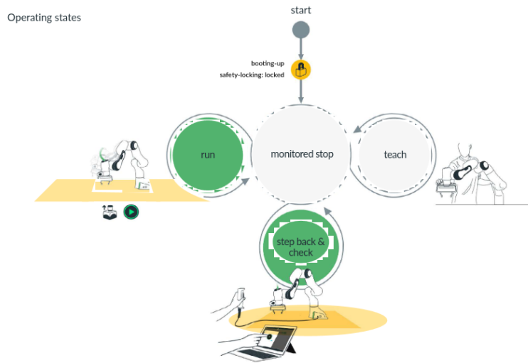
FIGURE II.1.32 – Fonctionnement du mode apprentissage pour le bras robotique Panda. Source : FRANKA EMIKA ROBOT'S INSTRUCTION HANDBOOK
