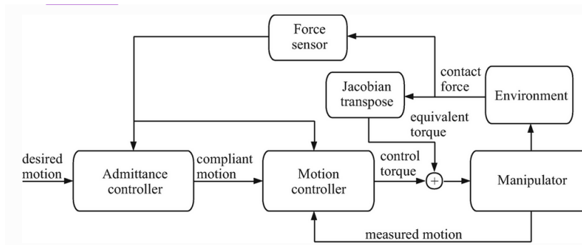
FIGURE II.1.19 – Schema qui illustre le fonctionnement de l'admittance. Source : le livre[0]
