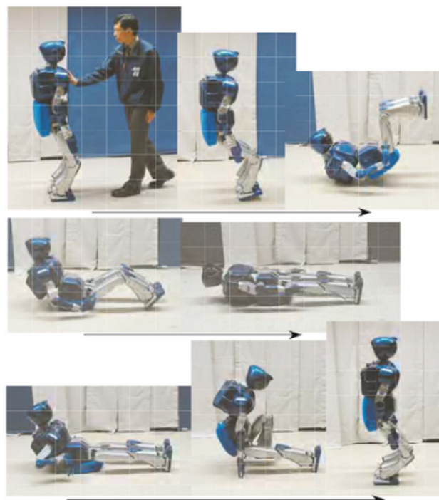
FIGURE II.1.24 – Illustration des mouvements pour se redresser de la chute. Source : le livre [8]
